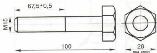
Рис. 2.3. Чертеж болта
